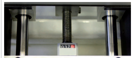
Rankinis reguliavimo ratukas su skaitmenine matavimo skale greitam ir tiksliam gręžimo stalo nustatymui
