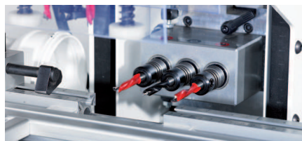
Gręžimo gylio ribotuvas su matavimo skale lengvam ir tiksliam gręžimo pozicijos nusistatymui
